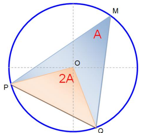
L'angle 2A est toujours le double de l'angle A
